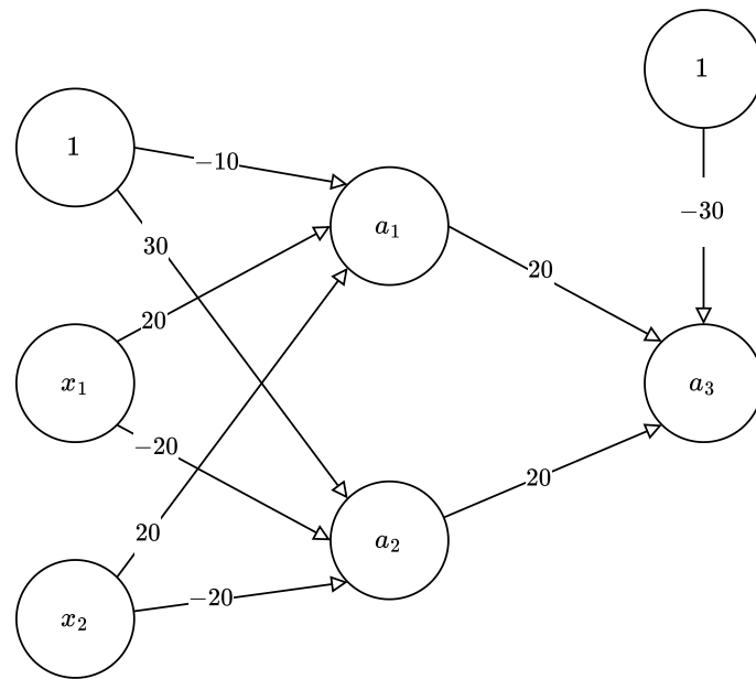
Figura 2.5: Rete di perceptroni per computare lo XOR
